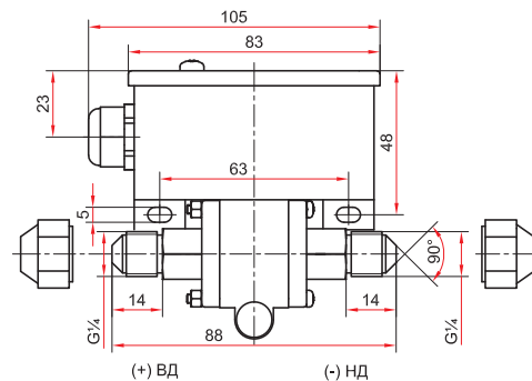
РДД-2Р с наружной резьбой с накидной гайкой G¼
