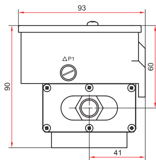
РДД-2Р с внутренней резьбой G¼
