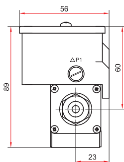
РДД-2Р с наружной резьбой с накидной гайкой G¼
