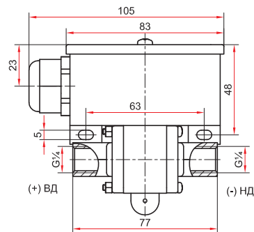
РДД-2Р с внутренней резьбой G¼
